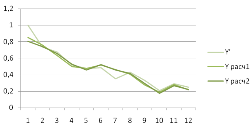
Рис. 1 – ЛММ
