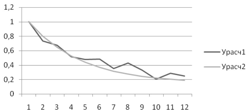
Рис. 2 – Авторегрессионная модель
