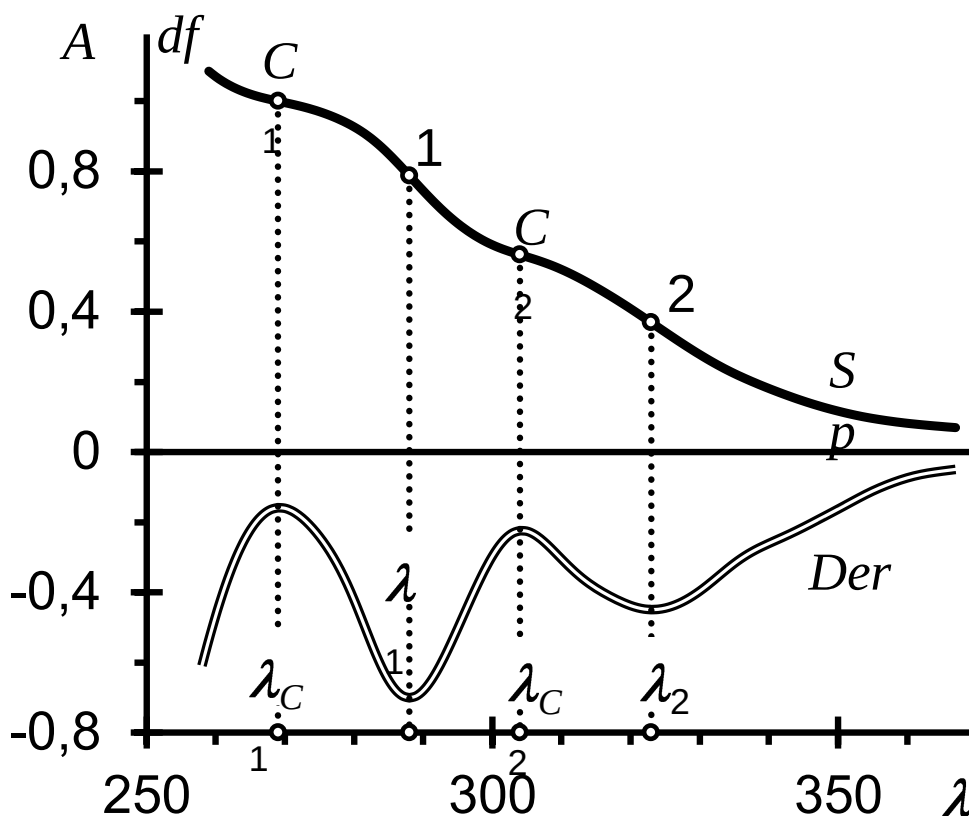
Рис. 3. Монотонный абсорбционный спектр ( Sp ) настойки корней аконита Кузнецова и производная ( Der ) спектра. C1 , C2 и \lambda_{C1} , \lambda_{C2} – ступеньки и соответствующие им длины волн. Другие обозначения см. на рис. 2
