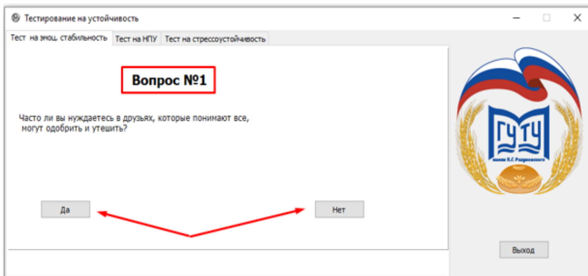
Рис. 1. Интерфейс программы
